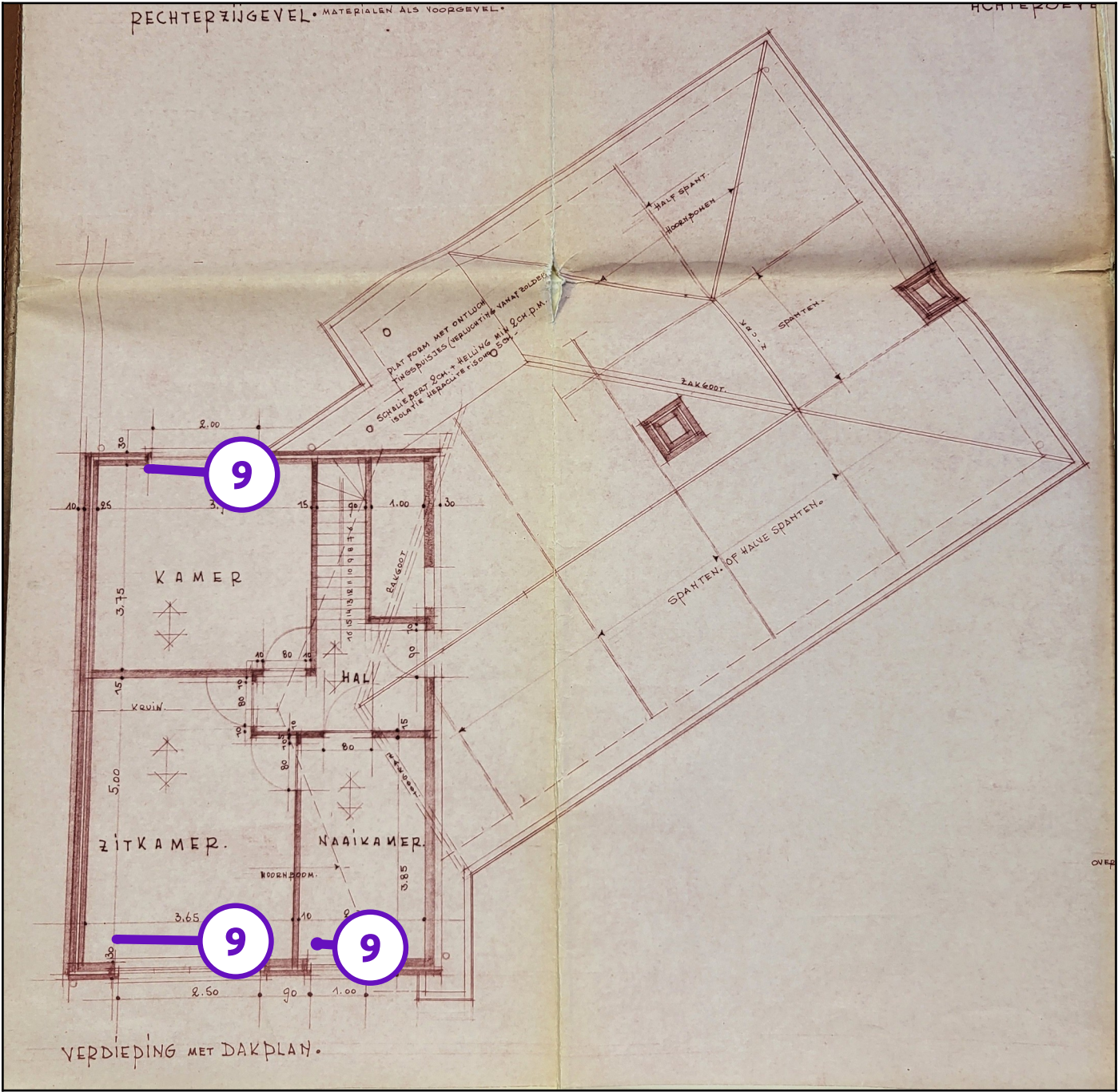
Legende van plan 1.13: VERDIEPING -ZOLDER
