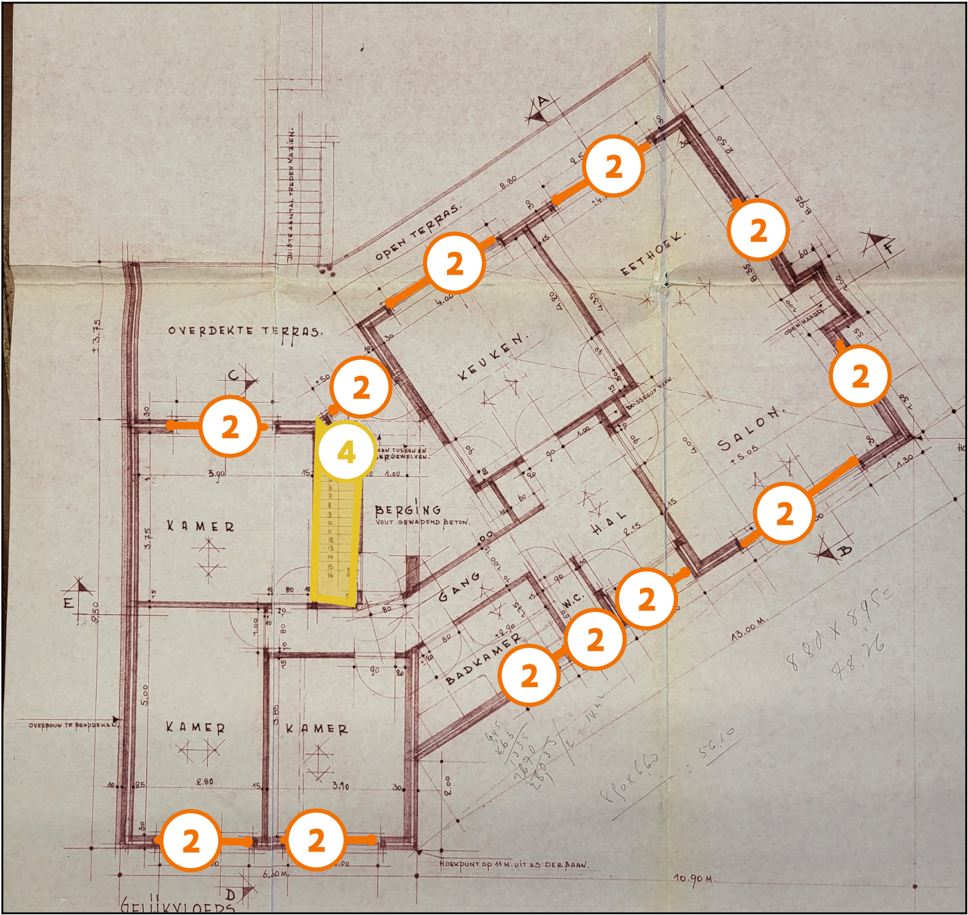
Legende van plan 1.7: GELIJKVLOERS
