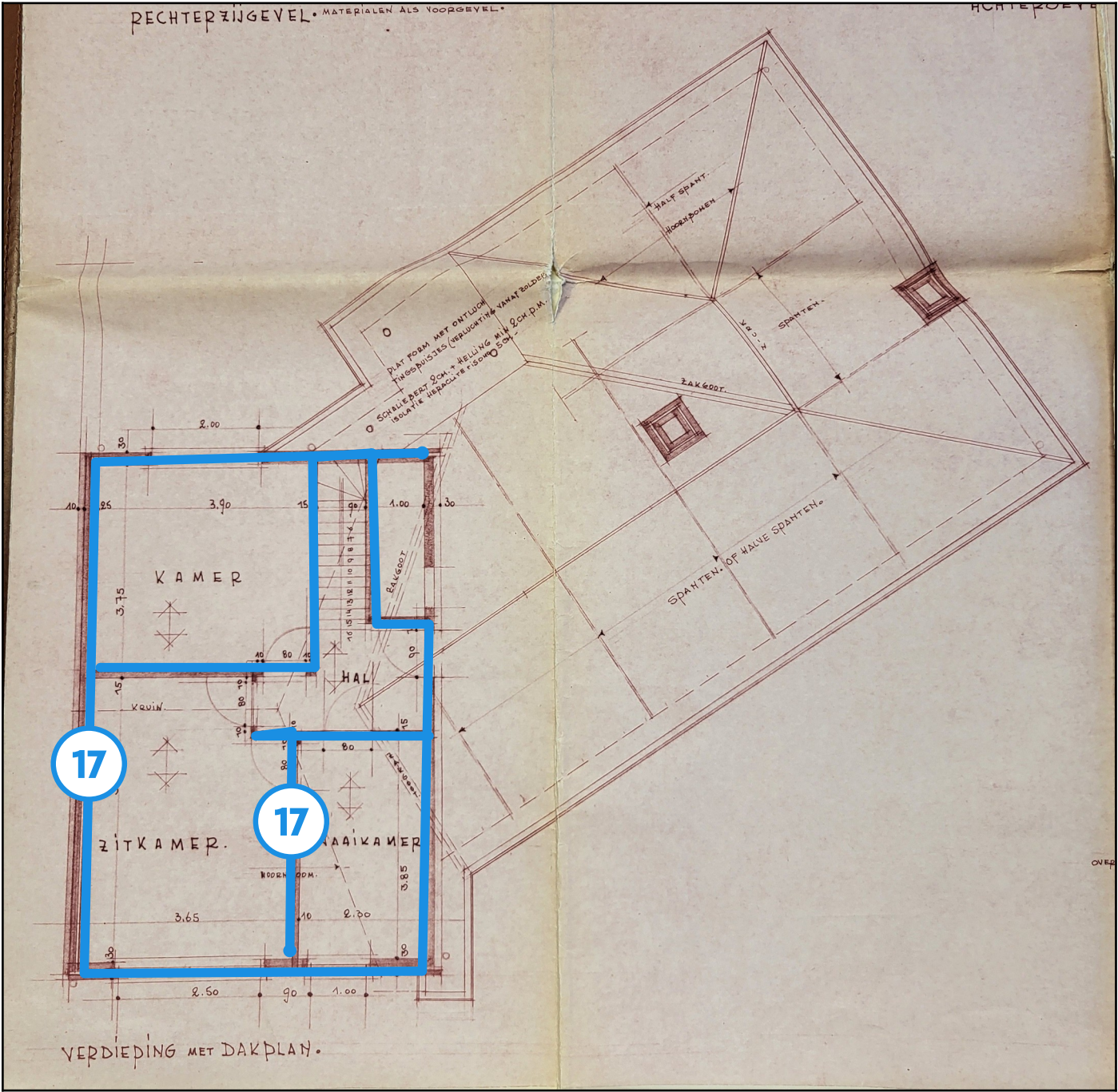
Legende van plan 1.11: VERDIEPING -ZOLDER
