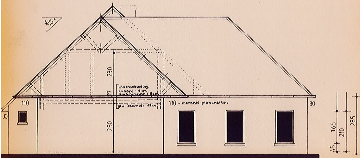
.zuidoostgevel.
