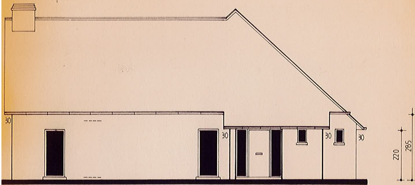
.noordwestgevel.
