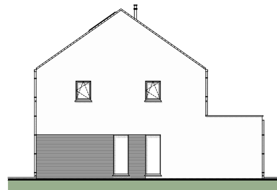
RECHTERGEVEL (Lot 4)
