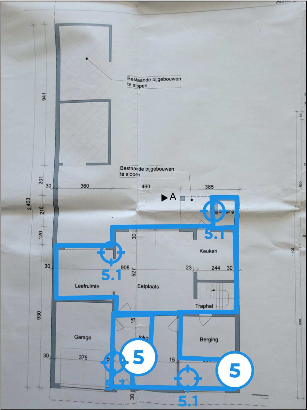
Legende van plan 1.3: Grondplan gelijkvloers
