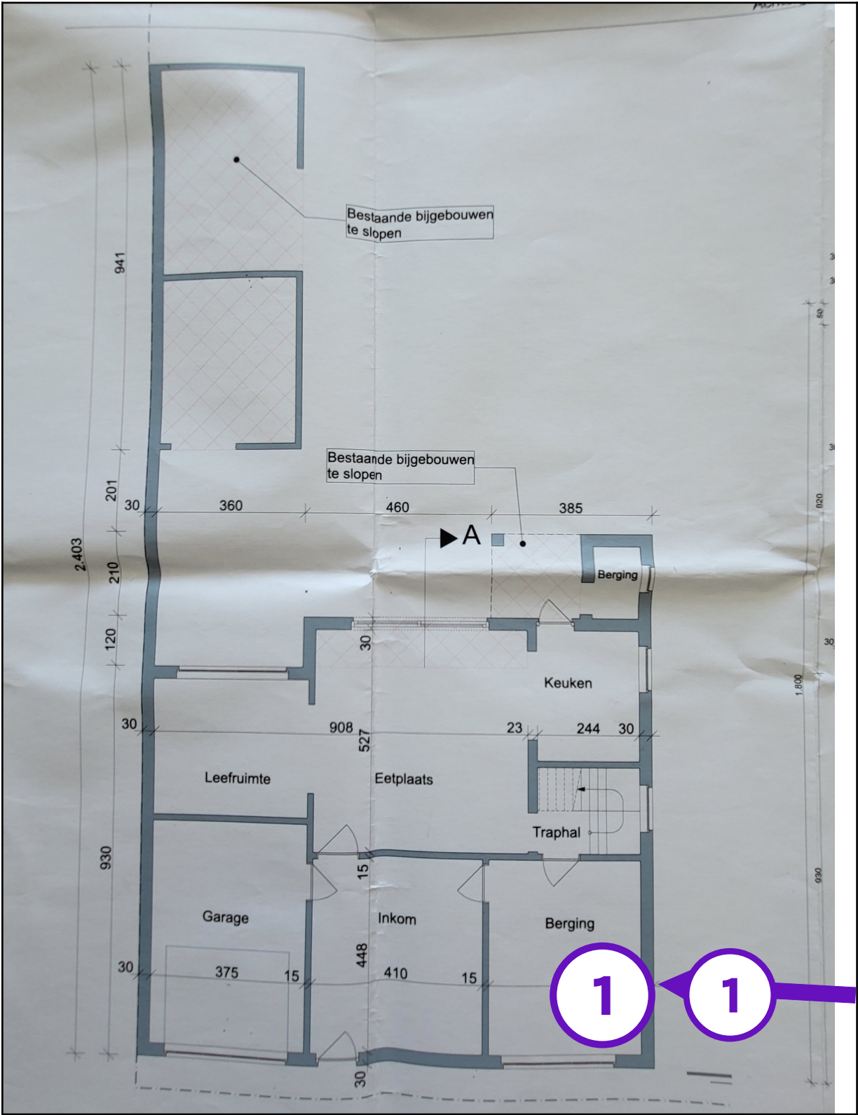
Legende van plan 1.10: Grondplan gelijkvloers
